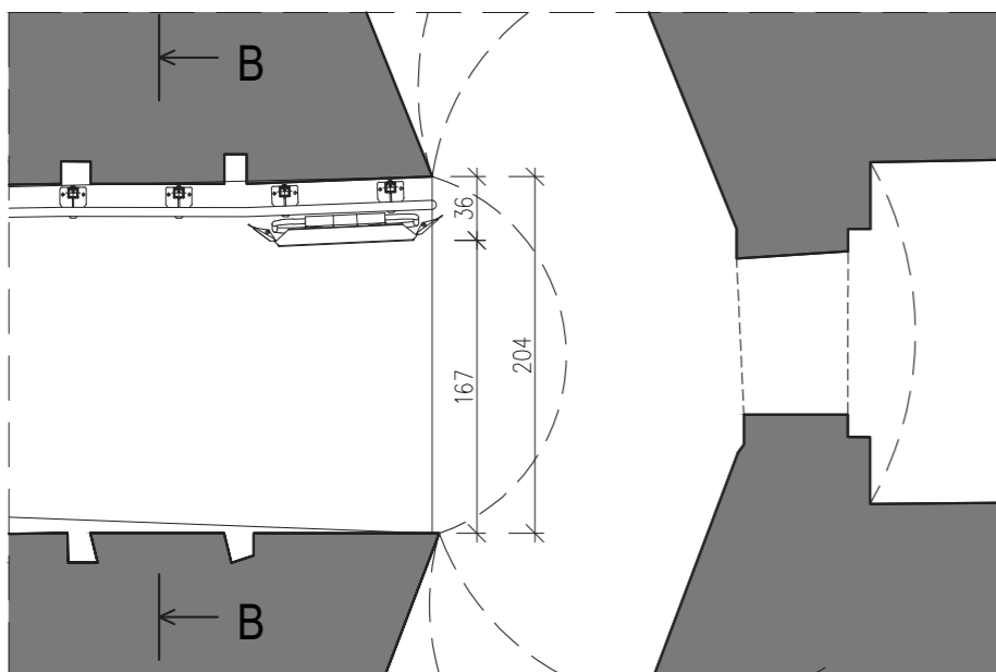
DETAL A
