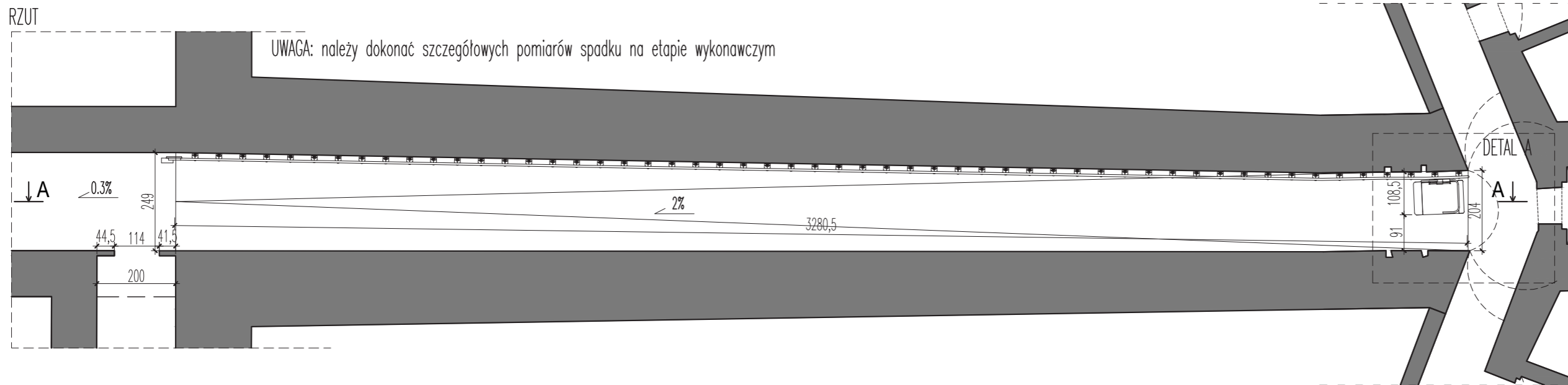
PRZEKRÓJ A-A
