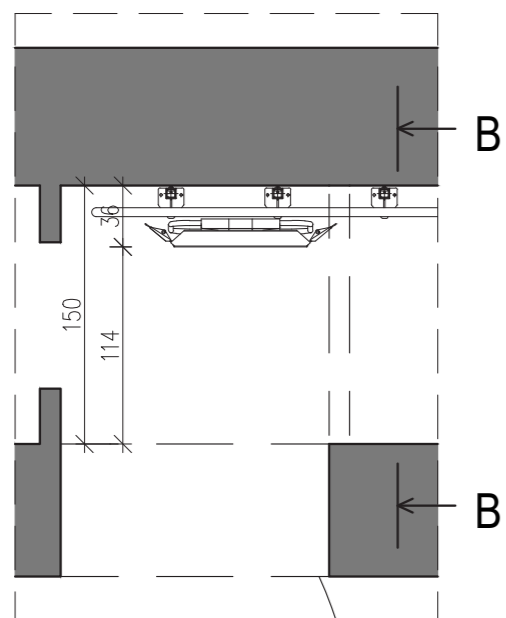
DETAL A
