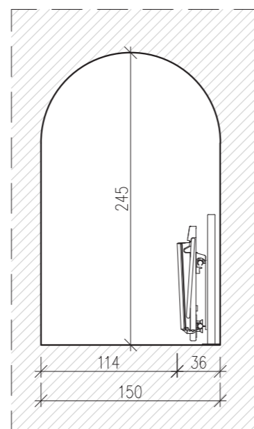
PRZEKRÓJ B-B
