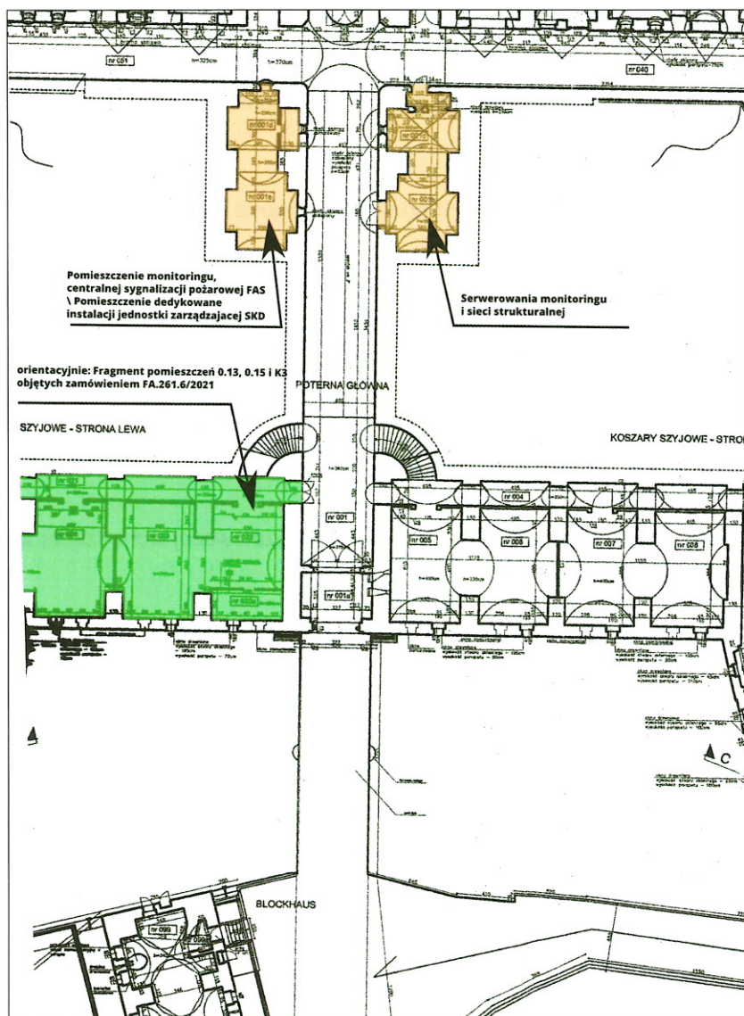
Rysunek 1 Orientacyjna lokalizacja pomieszczeń serwerowni oraz centrum monitoringu, centralnej sygnalizacji pożarowej, sieci strukturalnej i pomieszczeń dedykowanej lokalizacji instalacji jednostki zarządzającej SKD
